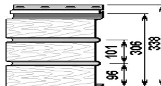
Соффит Т4
